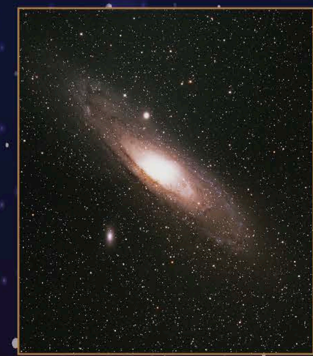
アンドロメダ銀河
